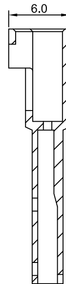
SECTION A-A
